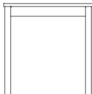
Parsons Table (K/D) 2710A07A15 W 30 D 30 H 30 1/2 (W 760mm D 760mm H 775mm)
